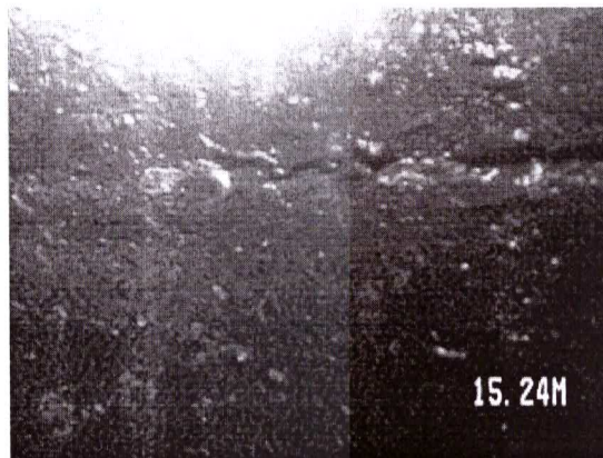
FOTOGRAMA 03 - Visada lateral mostrando uma solda aos 15,24 metros.
